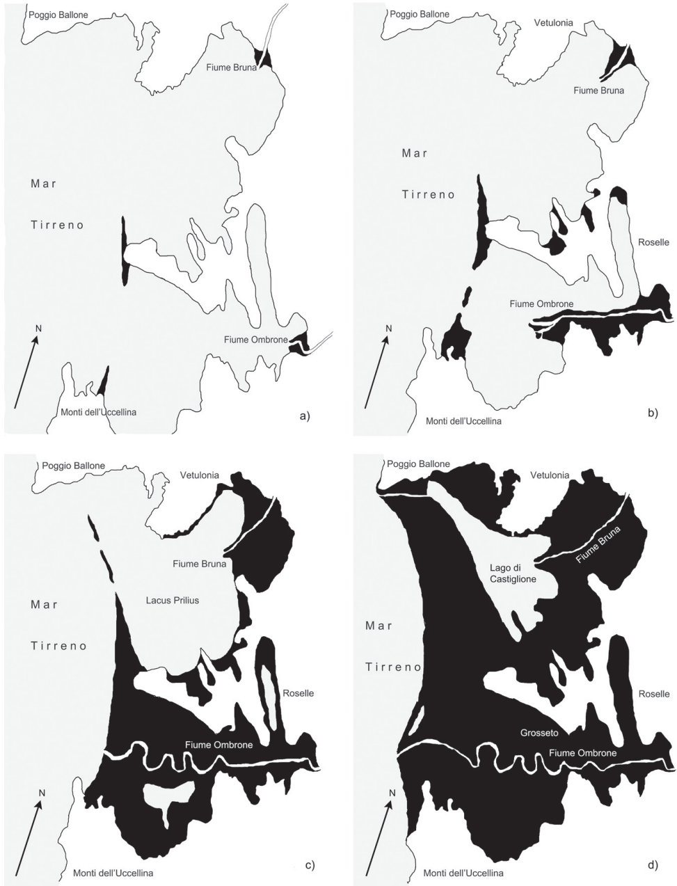
fig. 31 La piana di Grosseto. Evoluzione paleogeografica dell'area alla foce del fiume Ombrone. In bianco i canali fluviali e le aree emerse, in grigio le aree sommerse, in nero i depositi litorali e di colmamento delle lagune: a) circa 6000 anni fa; b) circa 3000 anni fa; c) fine del periodo romano; d) XIX secolo (da P. Bellotti, 2001, rielaborazione grafica a cura dell'Autrice).
