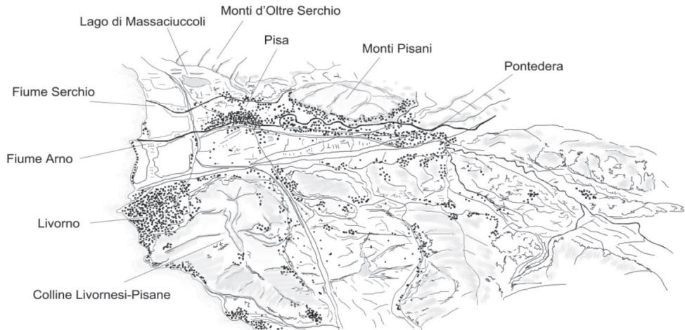
fig. 36 Rappresentazione prospettica a “volo d’uccello”, vista da SE, del territorio livornese e pisano. In primo piano le colline Livornesi-Pisane e la città portuale di Livorno. Sullo sfondo la pianura pisana contornata dai Monti Pisani e dai Monti d’Oltre Serchio e l’abitato della città di Pisa solcata dal fiume Arno che prosegue sino alla foce per gettarsi nel Tirreno. A nord di Pisa il corso del fiume Serchio che corre lungo la piana per poi sfociare anch’esso nel Tirreno (elaborazione grafica a cura dell’Autrice).
